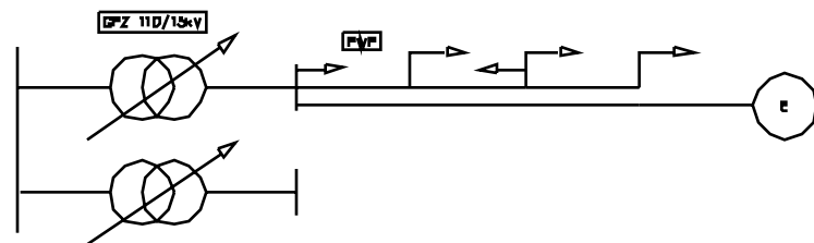
Możliwe warianty przyłączenia siłowni wiatrowych
